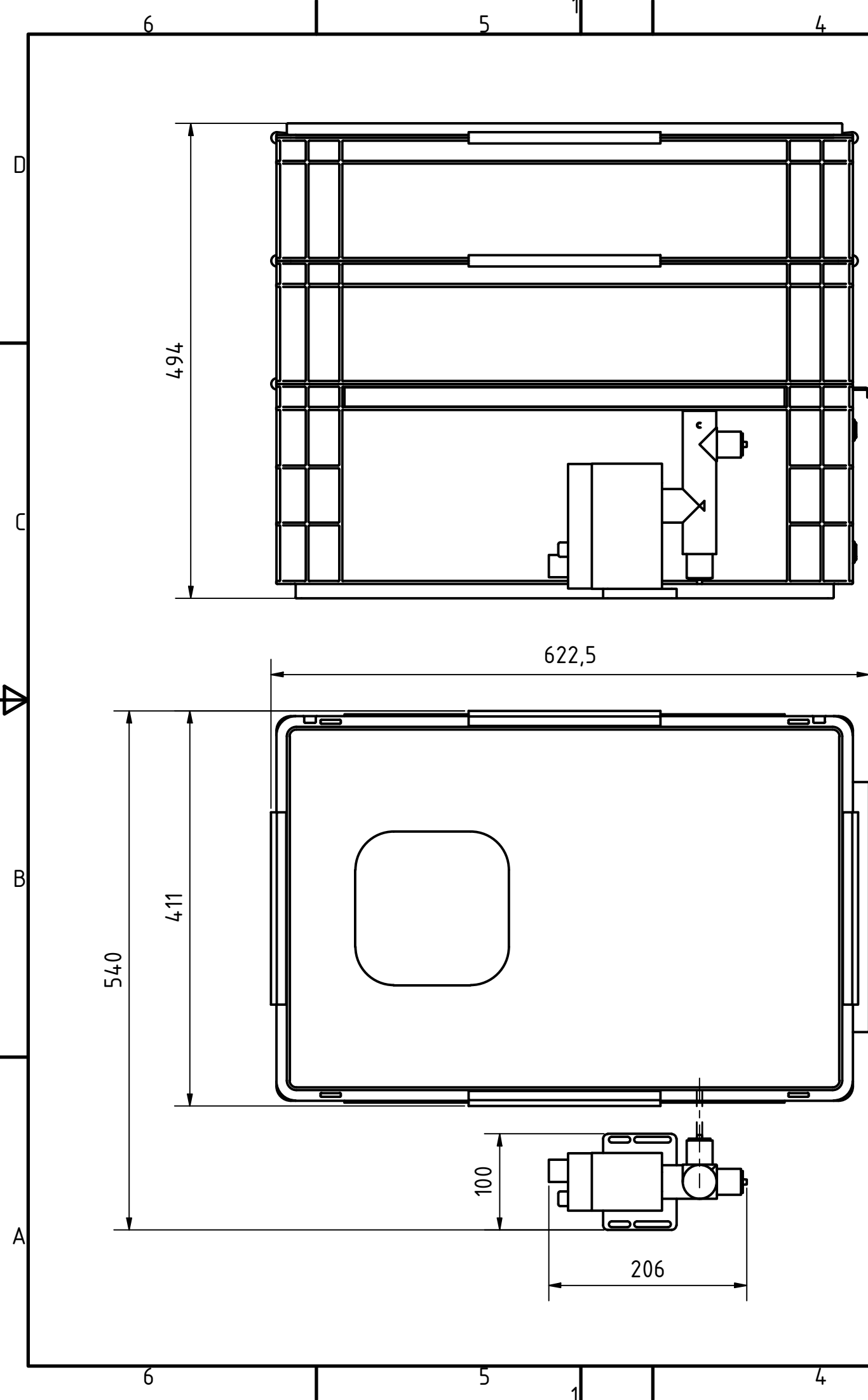
Kistenkaskade 70 Liter
